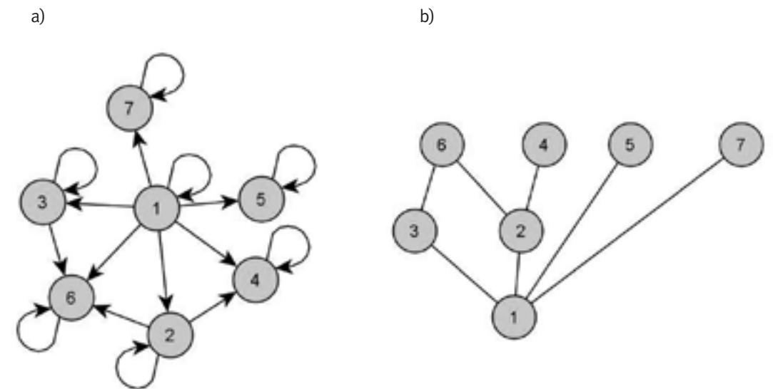
Rysunek 11. Reprezentacja relacji (20): a) graf relacji, b) diagram Hassego
